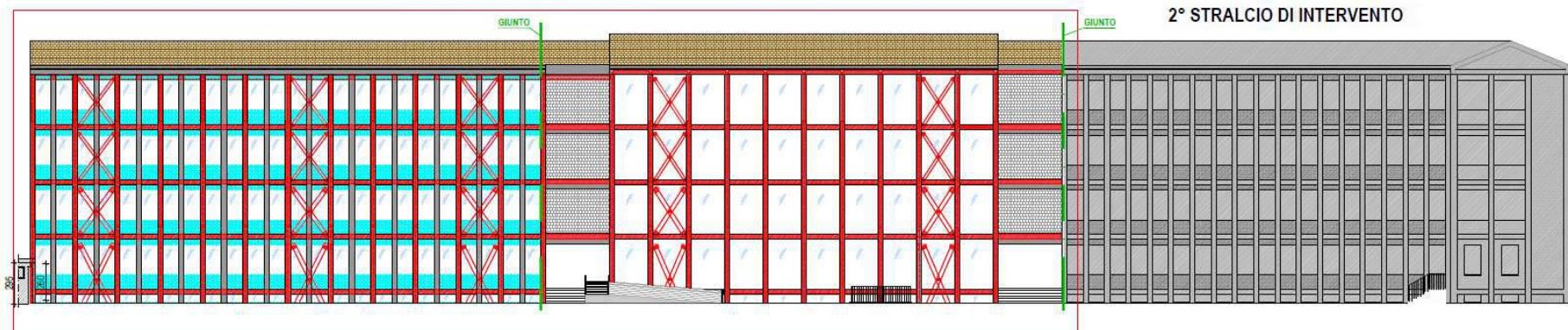
PROSPETTO "A" SCALA 1:200
